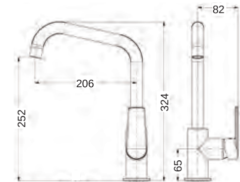
142515-100 Klint Chrome 150,00€ Περιστρεφόμενο ρουζούνι.
