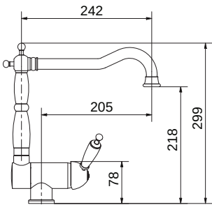
7596-100 Oxford Chrome 275,00€ Περιστρεφόμενο / Ανακλινόμενο ρουζούνι για χρήση παραθύρου. Ελάχιστο ύψος: 8 εκ.
