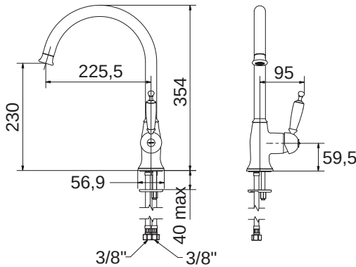
6381-400 Oxford Black matt 230,00€ Περιστρεφόμενο ρουζούνι.
