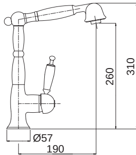
6388-400 Oxford Black matt 395,00€ Περιστρεφόμενο / αποσπώμενο τηλέφωνο με άθραυστο σπινάλι.
