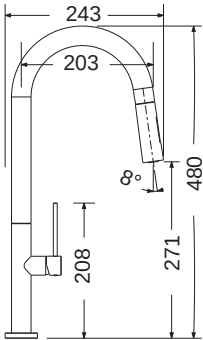
48780-100 Tozo Chrome 240,00€ Περιστρεφόμενο ρουζούνι με συρόμενο ντους 2πλής ροής (shower/spray).
