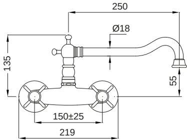
852-100 Princeton Chrome 250,00€ Τοίχου με περιστρεφόμενο ρουζούνι.
