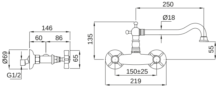
852-220 Princeton Bronze 295,00€ Περιστρεφόμενο ρουζούνι.
