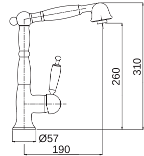
6388-100 Oxford Chrome 365,00€ Περιστρεφόμενο / αποσπώμενο τηλέφωνο με άθραυστο σπирάλ.
